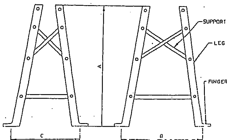
FIG. 11 STAND
